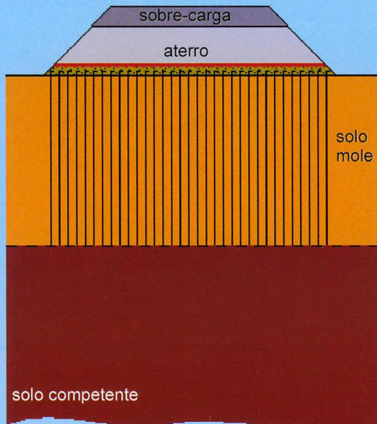
Figura 4 - Adensamento com drenos verticais
