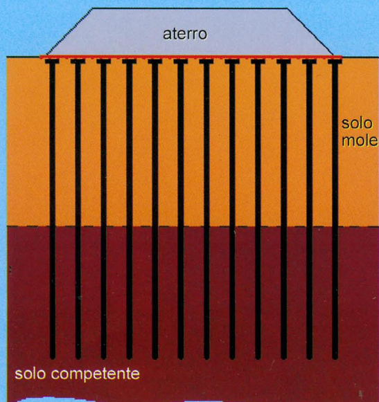
Figura 1 - Estruturação com estacas rígidas
