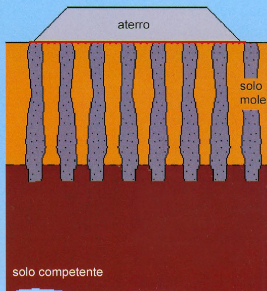
Figura 3 - Melhoria com colunas de brita
