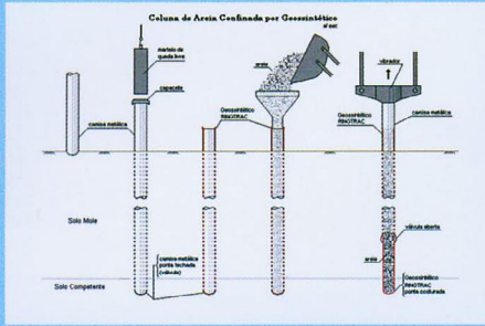
Figura 6 - Esquema da seqüência construtiva
